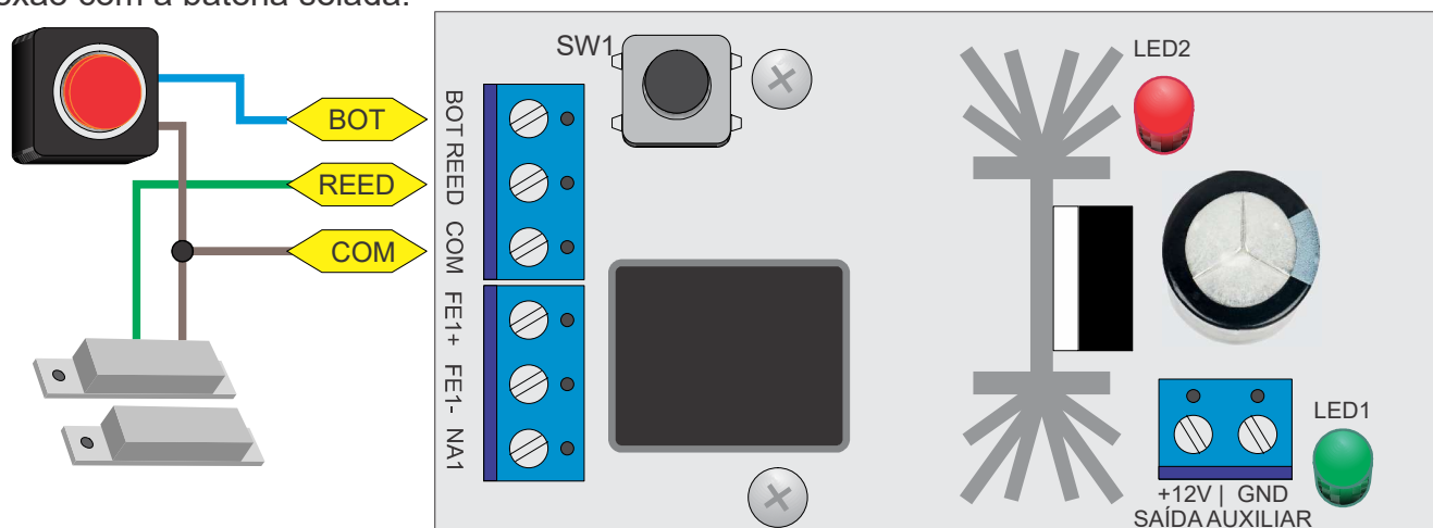
Figura 4 - Lado esquerdo da placa
