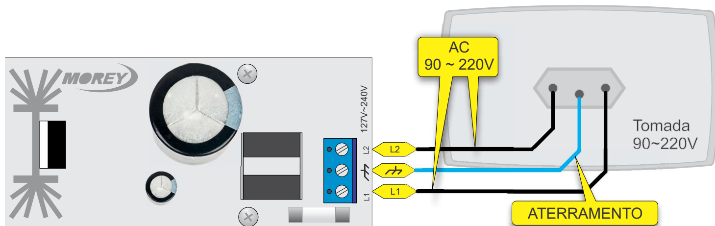
Figura 6 - Lado direito da placa
